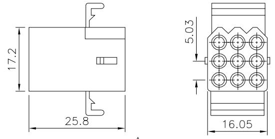
△ 3X03 Pin
