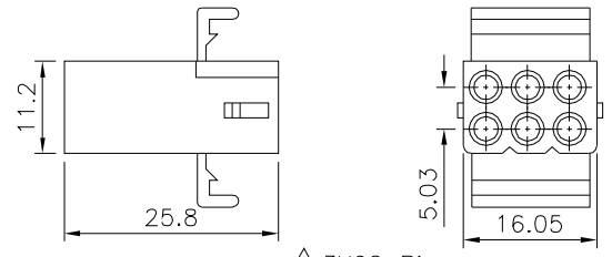
△ 3X02 Pin
