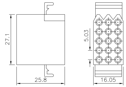
△ 3X05 Pin
