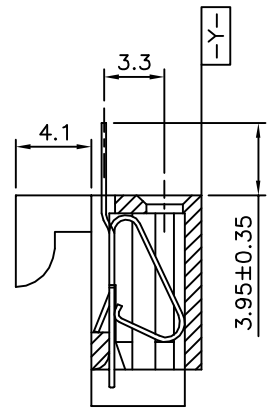
△△ Section:N-N
