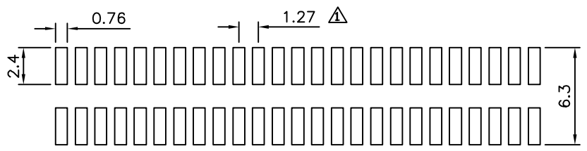
P.C.Board Layout
