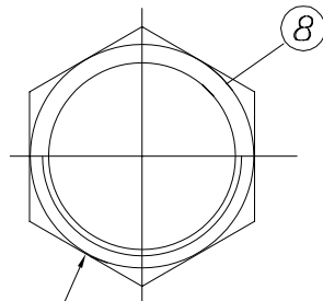
1/2-28UNEF-2B CLAMP NUT
