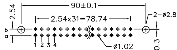
P.C.Board Layout
