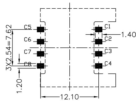
P.C.B LAYOUT(Tolerance:±0.05mm)
