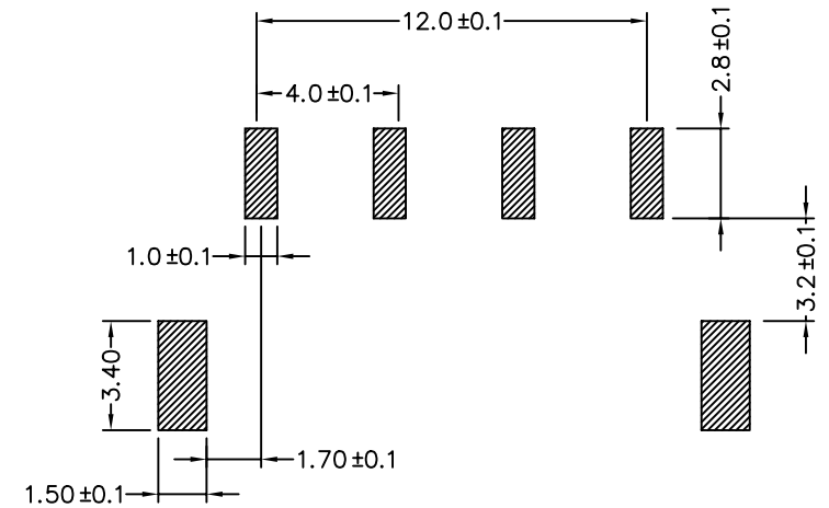
P.C.Board Layout
