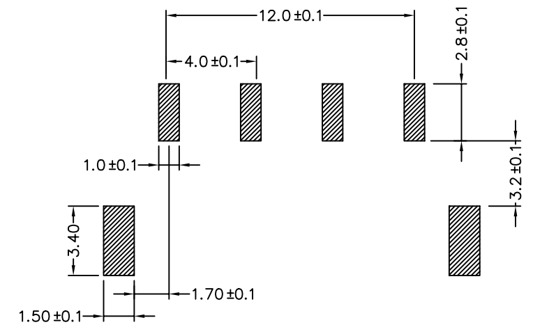
P.C.Board Layout
