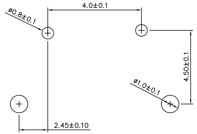
P.C.Board Layout
