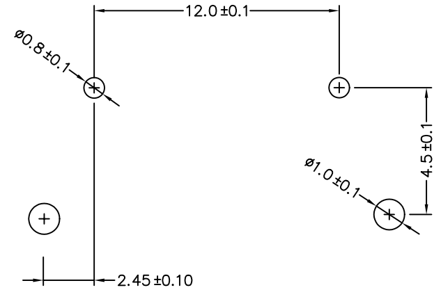
P.C.Board Layout
