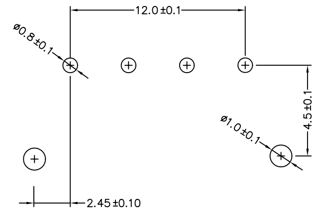
P.C.Board Layout
