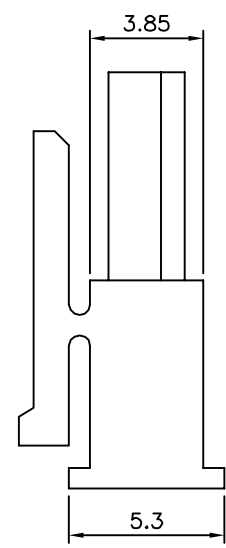
3~12 Pin
