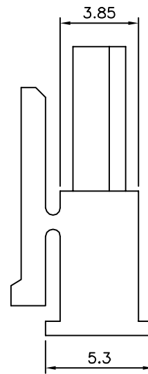
3~12 Pin
