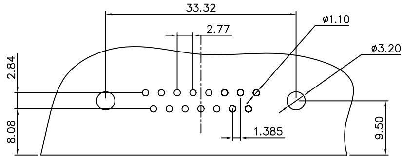
P.C.B EDGE RECOMMENDED P.C.B LAYOUT
