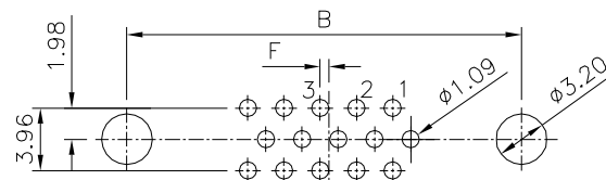
Recommended P.C.B. Layout(15 Pin)
