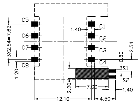
P.C.B LAYOUT(Tolerance: ±0.05mm)
