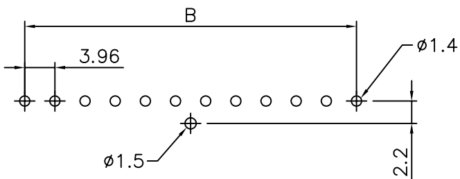
P.C.B Layout
