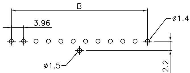
P.C.B Layout
