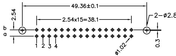
P.C.Board Layout
