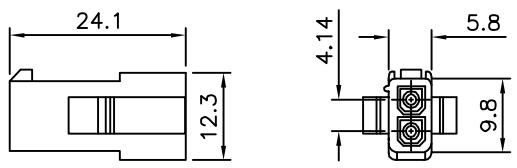
△ 1X02 Pin
