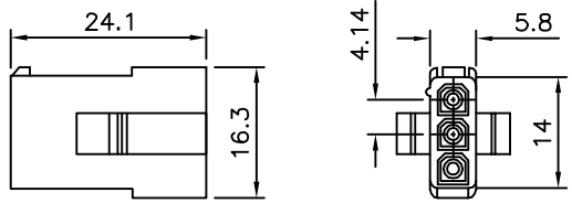
△ 1X03 Pin
