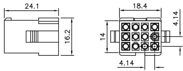
△△ 3X04 Pin
