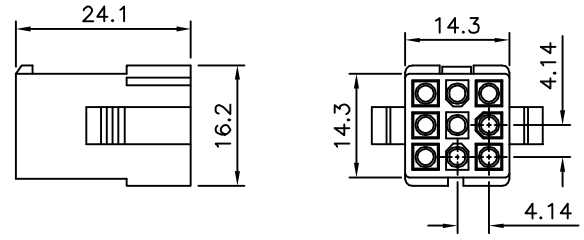
△ 3X03 Pin
