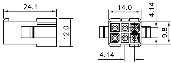
△ 2X03 Pin
