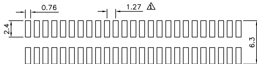
P.C.Board Layout
