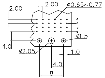
P.C.Board Layout
